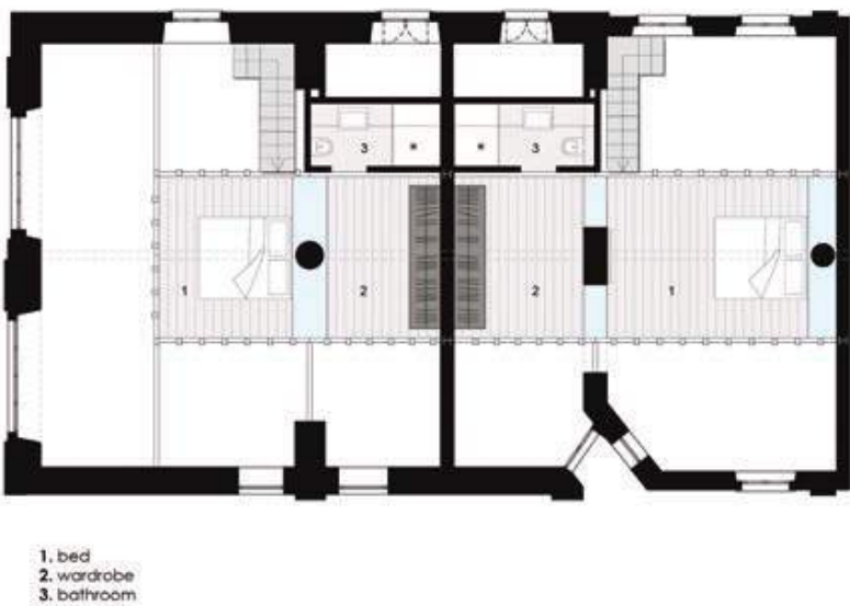
In alto, pianta piano terra e, sotto, pianta primo piano di Loft GO+JO. Qui accanto, Loft GO e, sopra, Loft JO, Milano.
